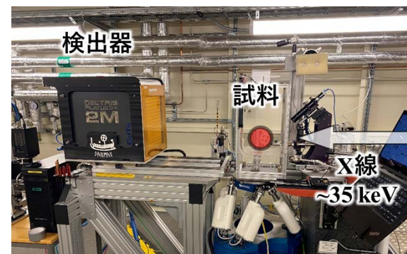
右側から左に向かってX線が入射、赤い丸で示した試料で回折したX線を左側の検出器で観測
