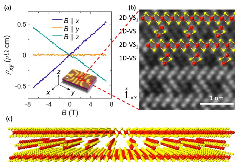
図1 異方性ホール効果を示す新しい超格子構造を発見。(a) 異方性ホール効果、(b) 2D-VS 2 /1D-VS 超格子構造の走査透過電子顕微鏡(STEM)による断面像。(c) 2D/1D ハイブリッド超格子のモデル図。
