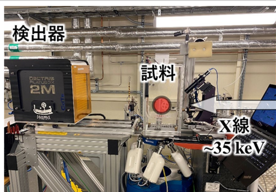
右側から左に向かって X 線が入射、赤い丸で示した試料で回折した X 線を左側の検出器で観測
