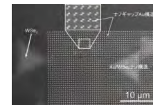
Au/WSe 2 ナノ構造の電子顕微鏡写真
